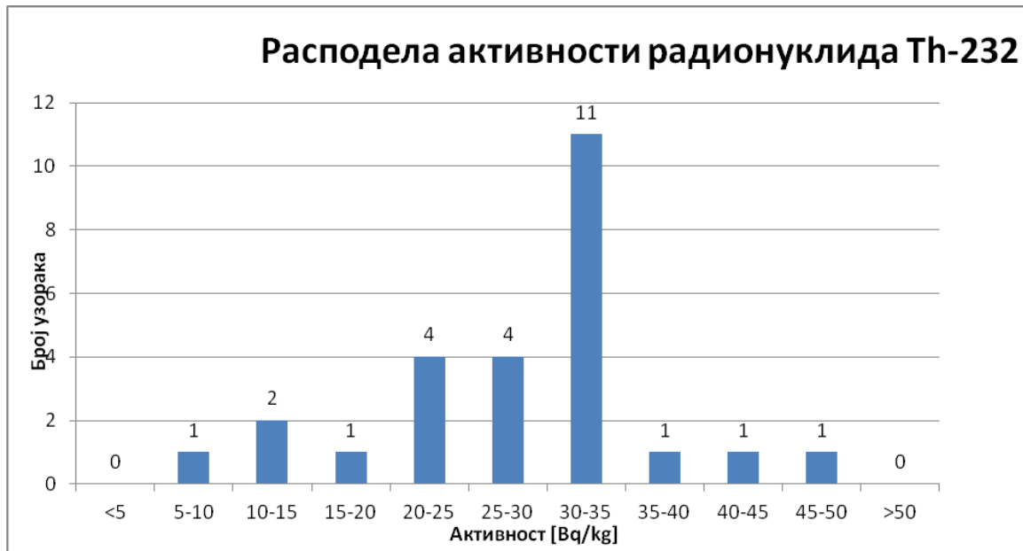
Слика 3. Расподела активности радионуклида ^{232}\text{Th}
