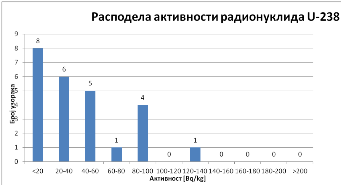
Слика 5. Расподела активности радионуклида ^{238}\text{U}
