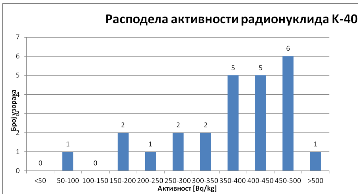
Слика 1. Расподела активности радионуклида ^{40}\text{K}
