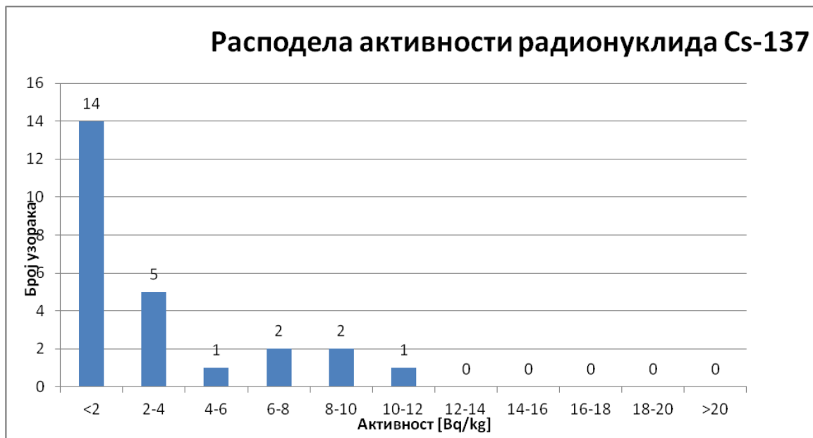
Слика 4. Расподела активности радионуклида ^{137}\text{Cs}
