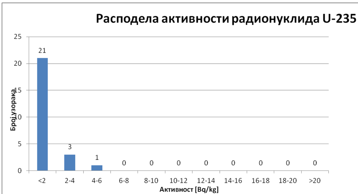
Слика 6. Расподела активности радионуклида ^{235}\text{U}
