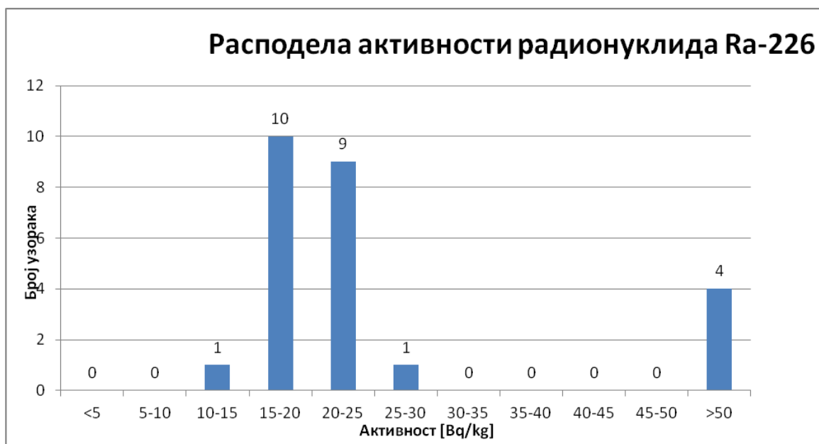
Слика 2. Расподела активности радионуклида ^{226}\text{Ra}
